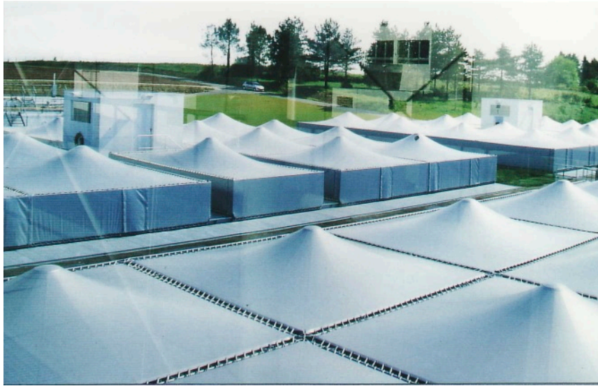
Couverture métallo-textile sur les bassins de décantation
